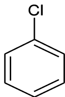
Chlorobenzene
